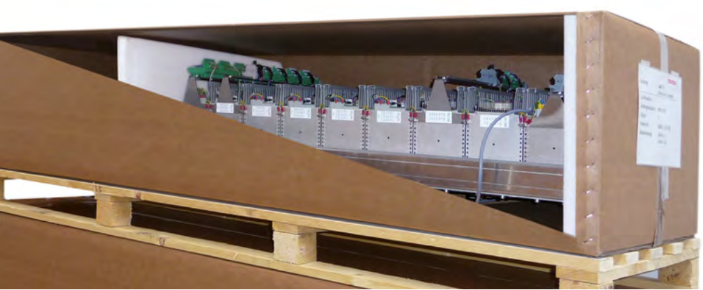
Gewichtsoptimierte Luftfrachtverpackung Schaltschrank
